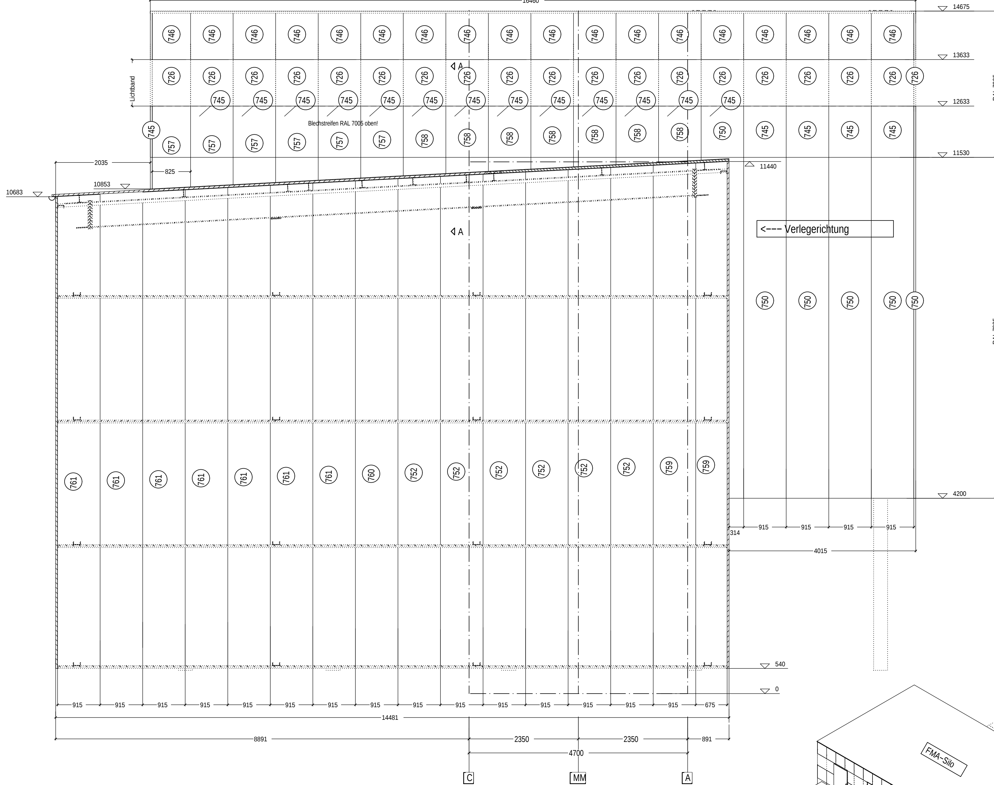
Ansicht Wand 4 – M. 1:50
