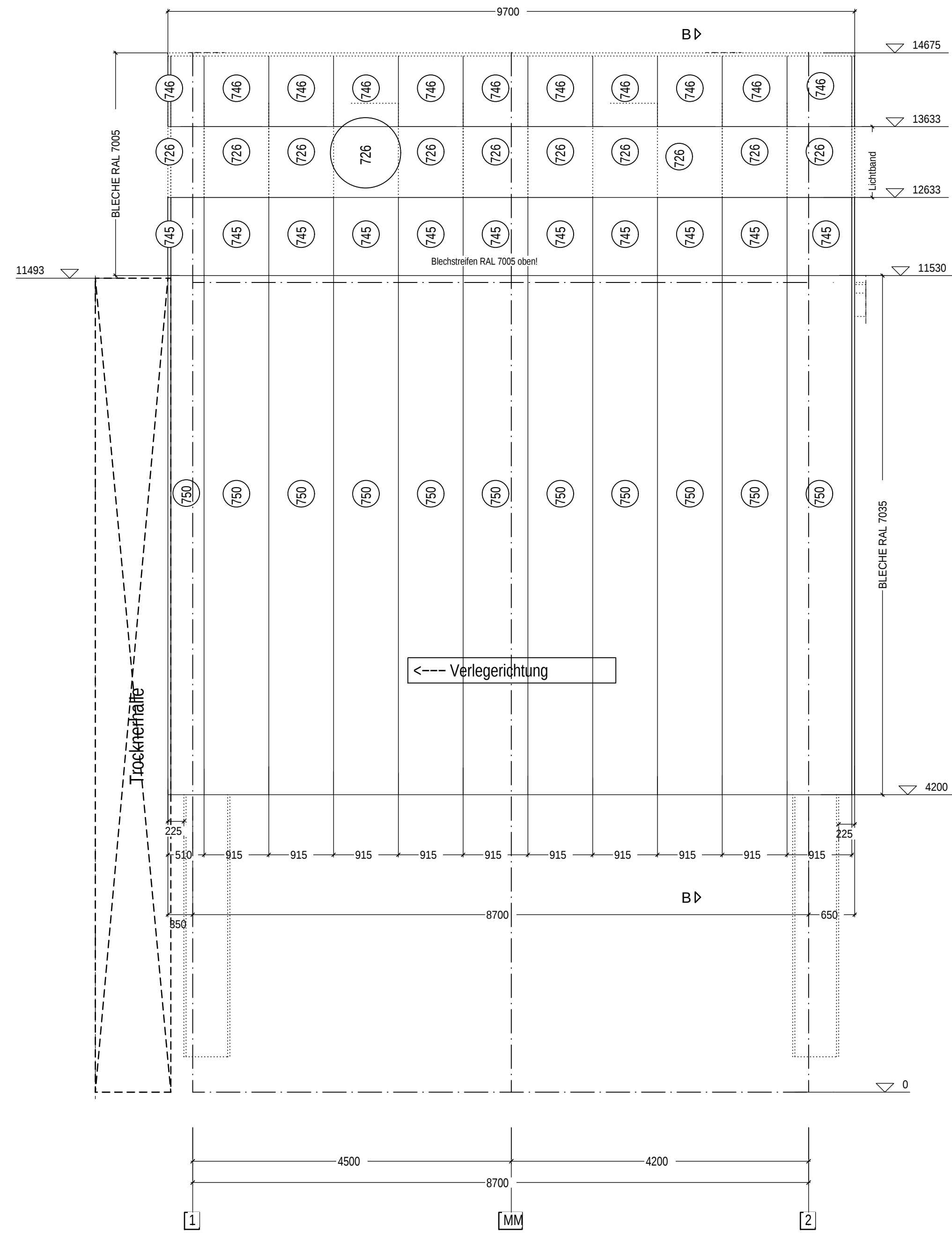
Ansicht Wand 3 – M. 1:50
