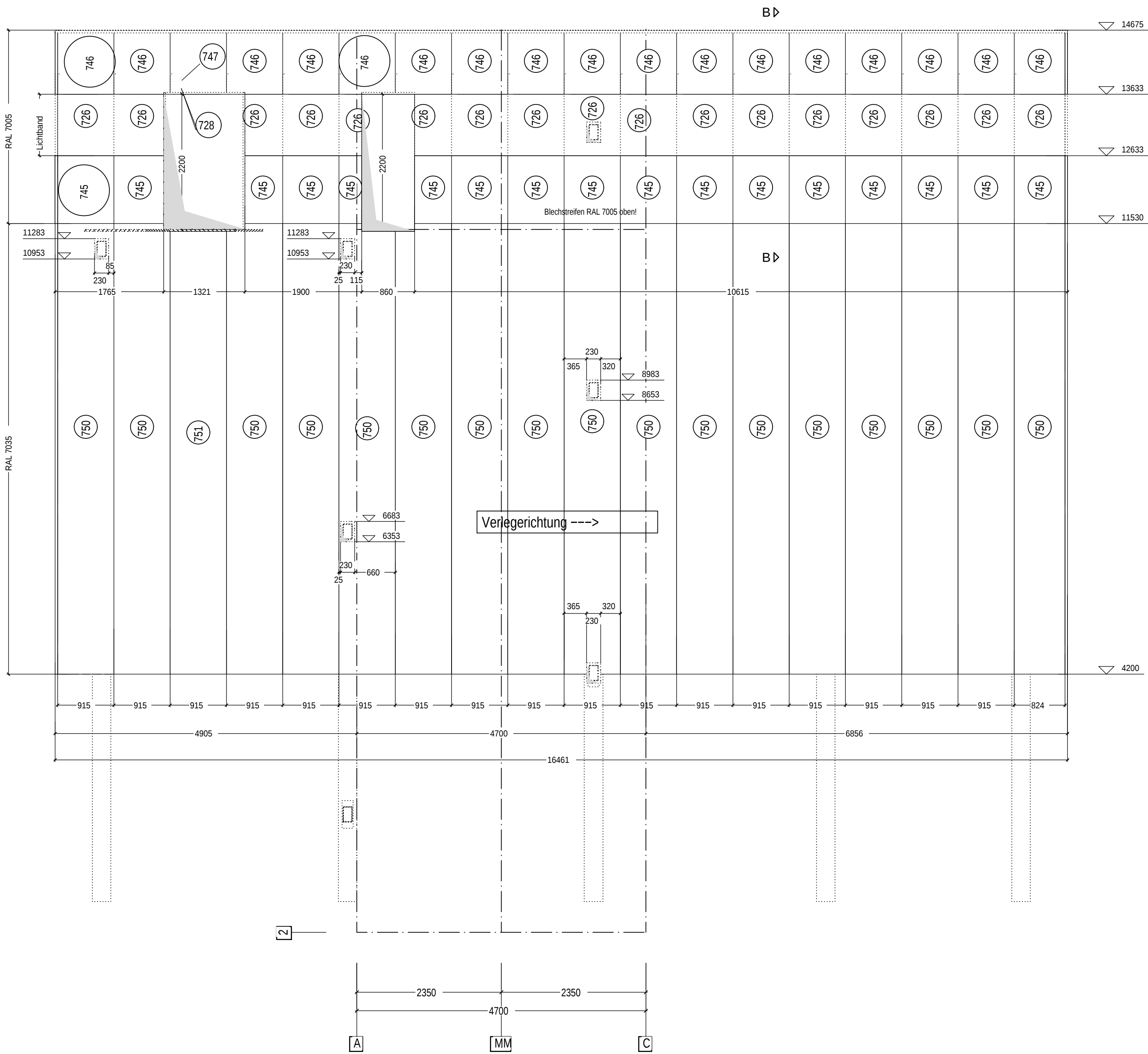
Ansicht Wand 2 – M. 1:50
