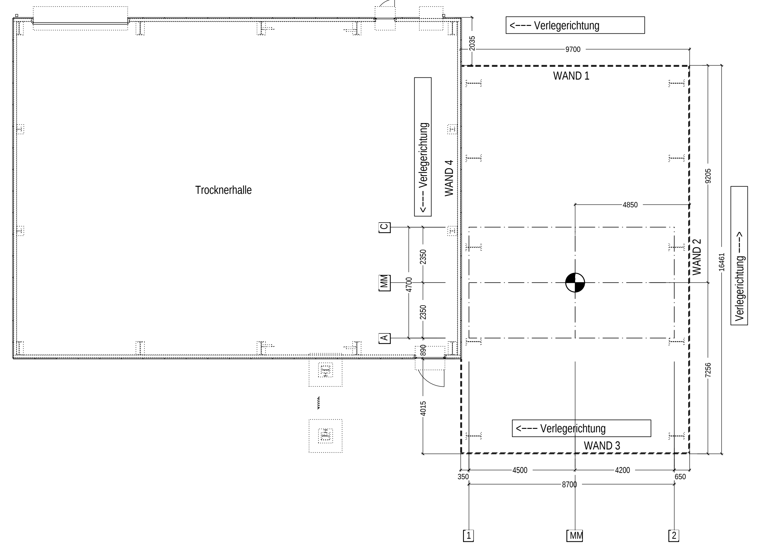
Grundriss FMA-Silo – M. 1:100
