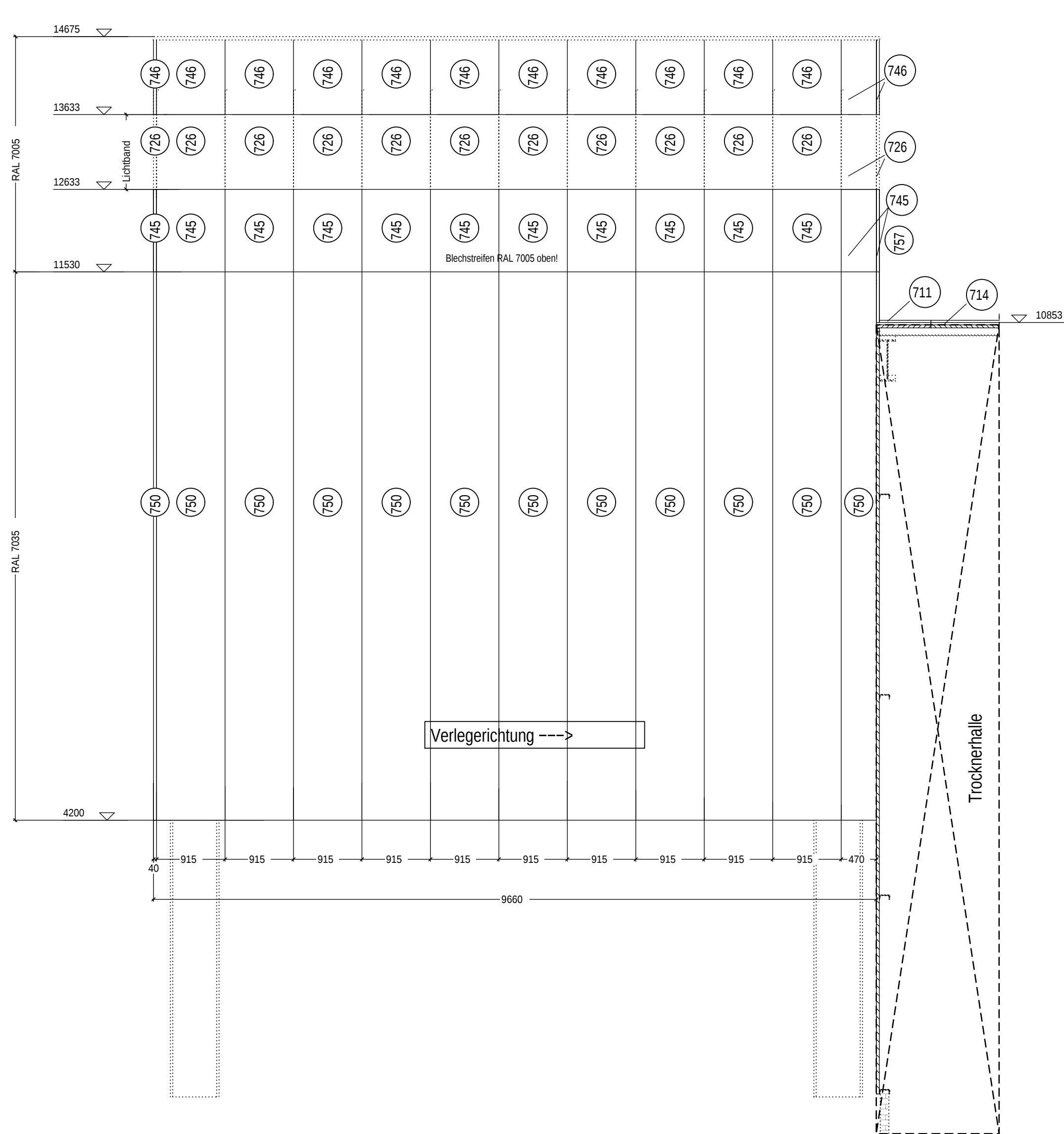
Ansicht Wand 1 – M. 1:50
